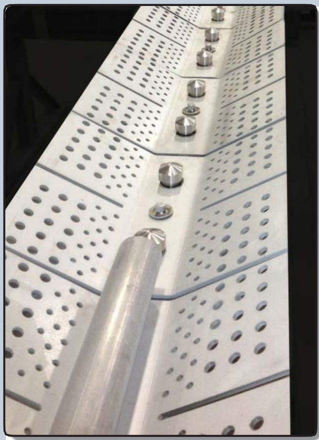
Канальная горелка с низким уровнем выбросов NOx
