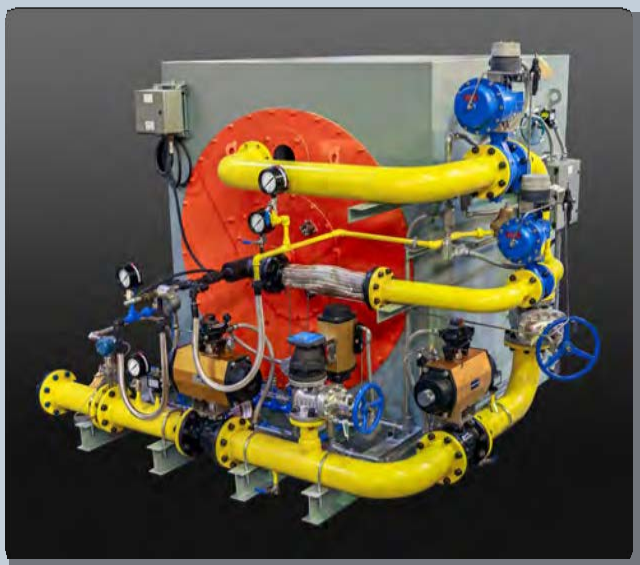
Горелка ZEECO GLSF Free Jet
