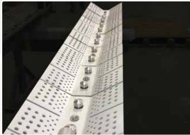
Канальная горелка с низким выбросом NOx
